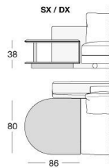
Accessori per elemento terminale / End unit accessories / Аксессуары для боковой секции
